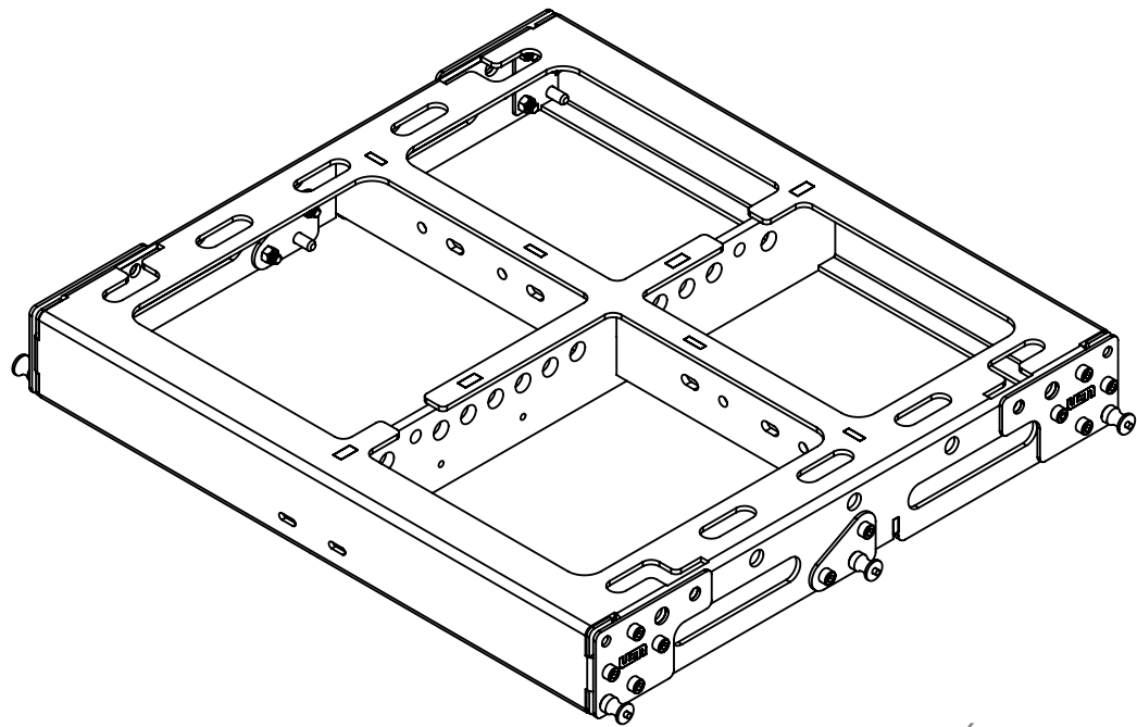
VISTA ISOMÉTRICA
